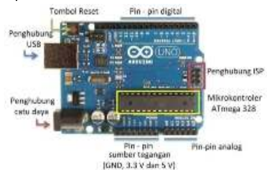
Gambar 6. Rangkaian Arduino Uno
